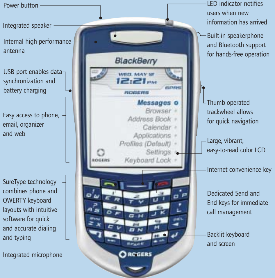
BlackBerry 7100r Shown Actual Size
